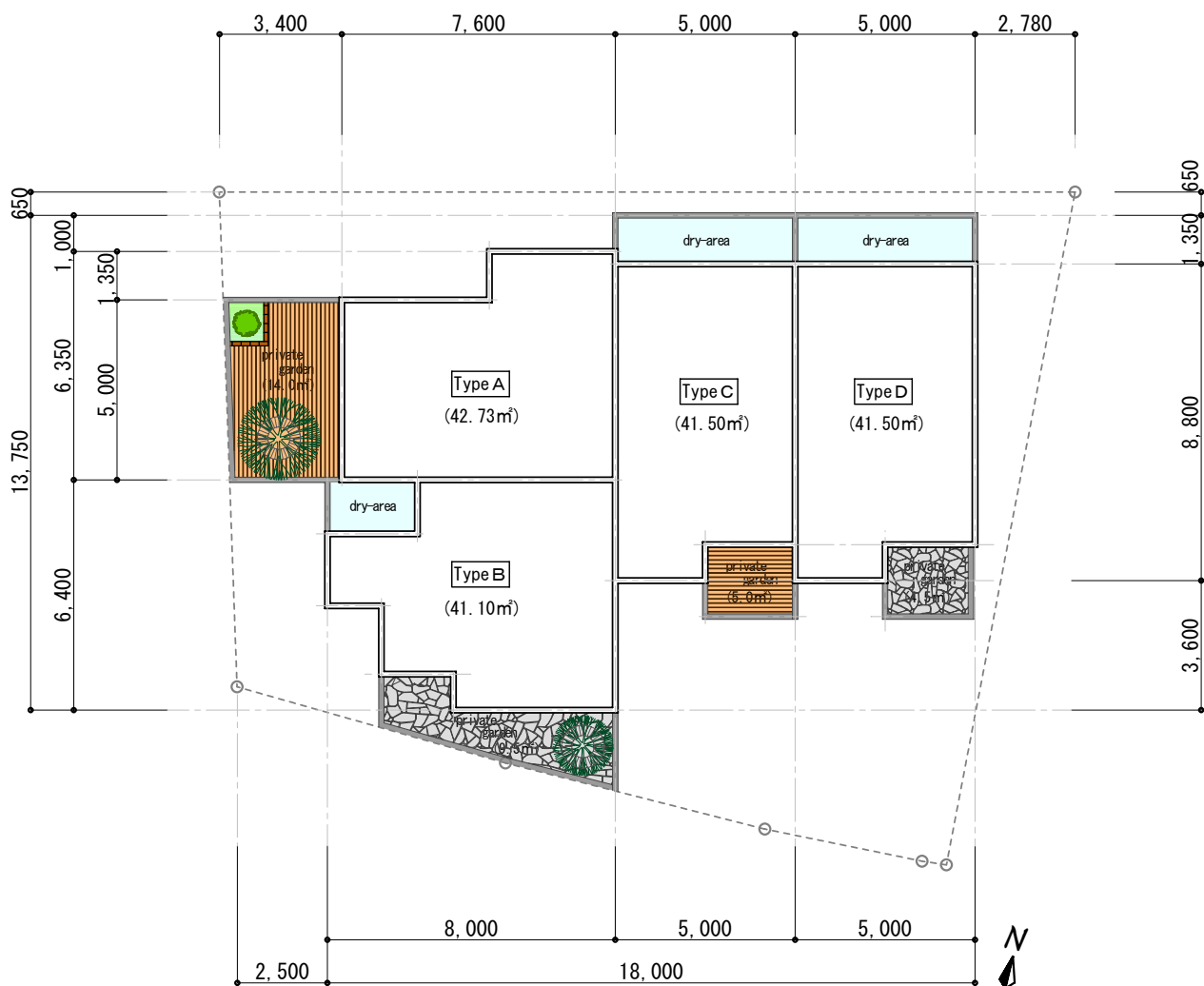
地下1階プラン S=1/200
